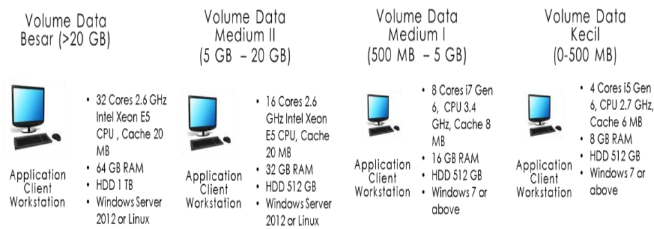
Gambar 4. Spesifikasi Perangkat Keras dan Perangkat Lunak untuk Pelaporan
